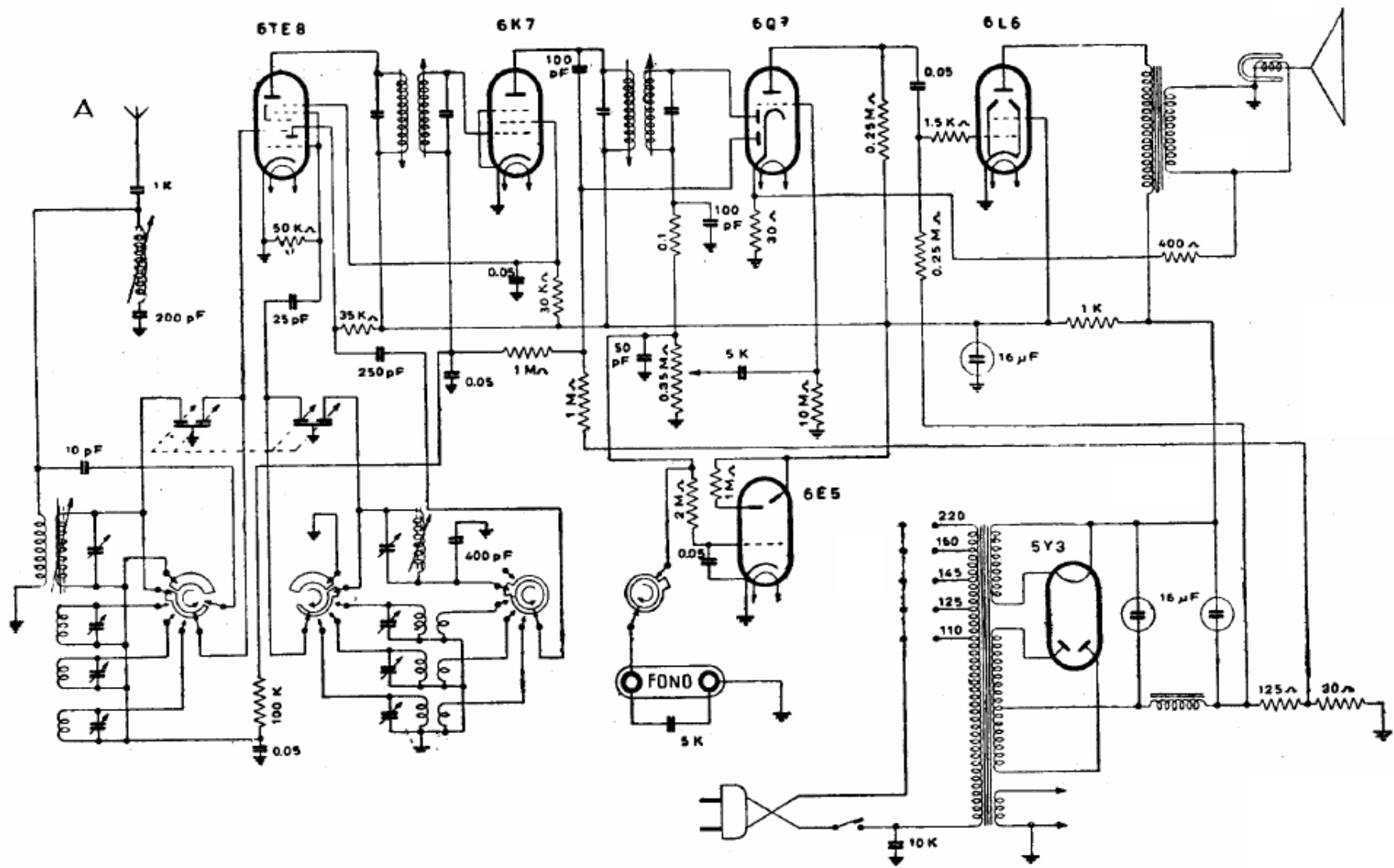
IRRADIO - Mod. AK 18 - Media frequenza 467 kc. Potenza d'uscita 4 watt. Consumo 55 watt.
